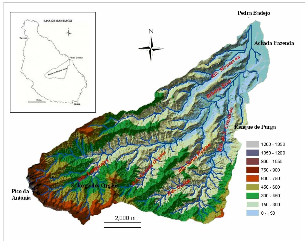
FIGURA 1 – Modelo Digital do Terreno da Bacia da Ribeira Seca (Costa e Nunes, 2007b).
