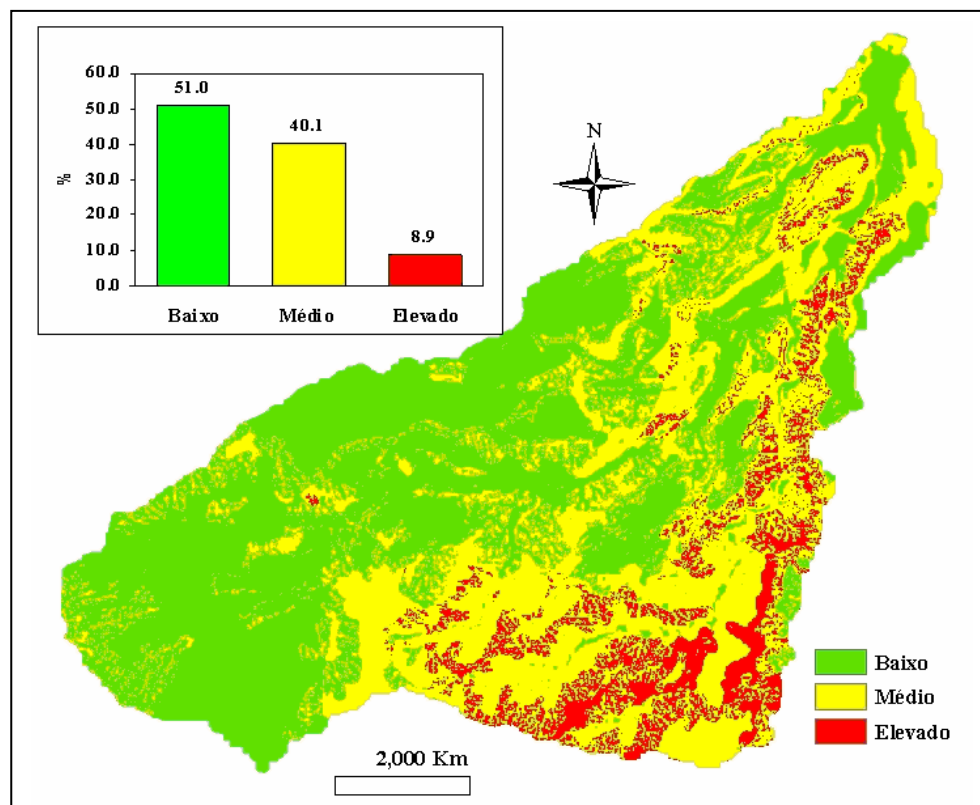
FIGURA 8 – Susceptibilidade à erosão hídrica em função de factores geomorfológicos, de coberto vegetal e de intensidade pluviométrica.
