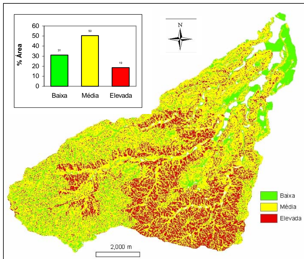
FIGURA 2 – Susceptibilidade à erosão hídrica em função de factores geomorfológicos na bacia da Ribeira Seca (Costa e Nunes, 2007b).
